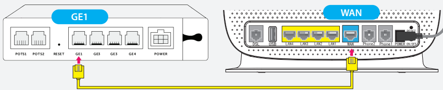
Bottom side of ONT box
